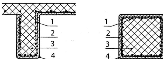
Рис.8.11. Восстановление железобетонных конструкций 1 – «старая» арматура; 2 – арматурная сетка; 3 – «здоровый» бетон; 4 – торкрет-бетон.
